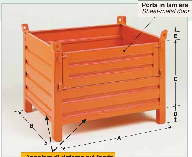
Angolare di rinforzo sul fondo Strengthening frame on bottom
